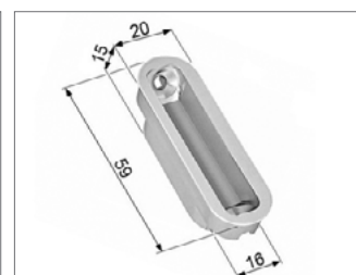
Minimal XT megfordítható műanyag zárólemez
