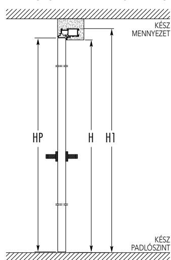
TOKSZERKEZET KERESZTTARTÓVAL
