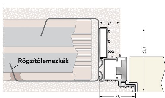
Tokszerkezet vakolt falhoz
