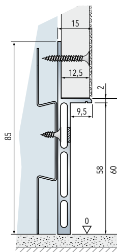
Egy gipszkarton lemezre szerelt szegélyléc
