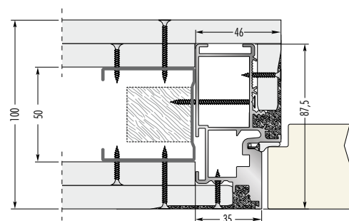
Tokszerkezet gipszkarton falhoz két lemezzel A kész fal vastagsága 100 mm
