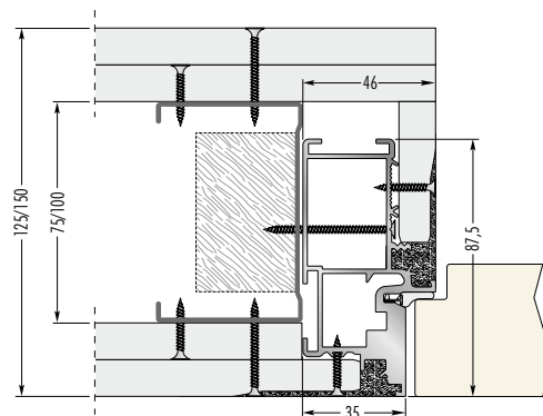
Tokszerkezet gipszkarton falhoz két lemezzel A kész fal vastagsága 125/150 mm
