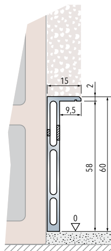
Épített falra szerelt szegélyléc
