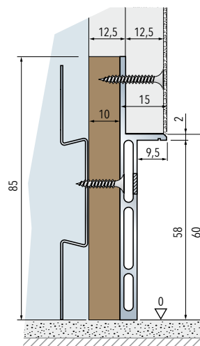
Gipszkarton falra szerelt szegélyléc dupla lemez
