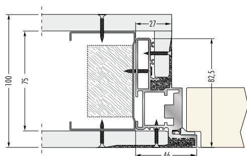
Tokszerkezet gipszkarton falhoz egy lemezzel A kész fal vastagsága 100 mm
