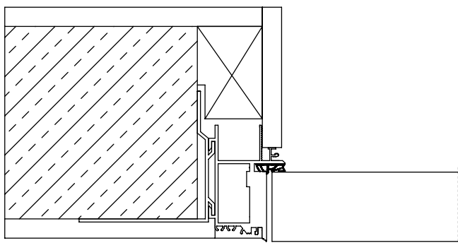
Falcolatlan ajtó vízszintes metszete
