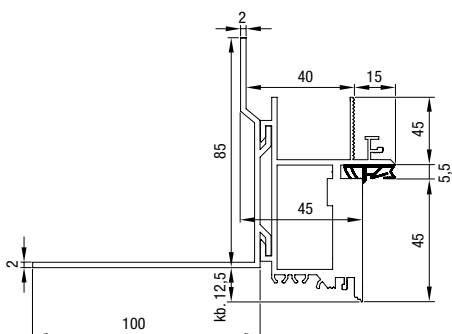
Zeroline tok méretezése
