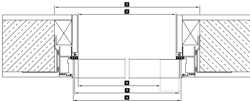
Falcolatlan ajtólap vízszintes metszete
