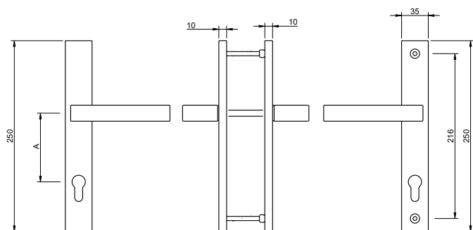
Puxador par de alta segurança Grau de resistência classe 3 Disponível versão fixo/móvel e móvel/móvel com muleta
