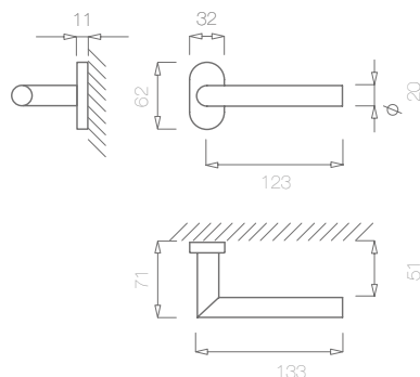
Puxador par para porta de alumínio- Espelho oval Mola recuperadora Ferro quadrado de 8x100mm Adaptador metálico
