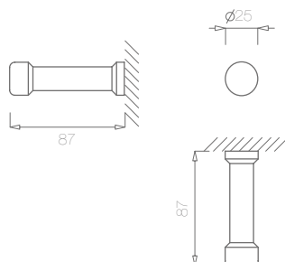
Batente limitador de porta Constituído por duas peças com rosca
