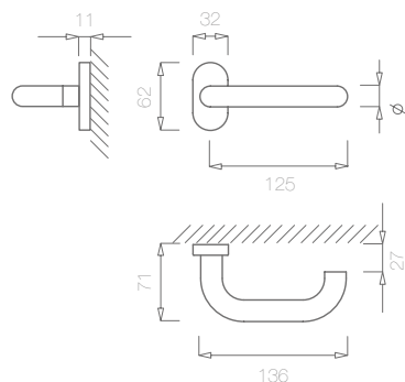
Puxador par para porta de alumínio- Espelho oval Mola recuperadora Ferro quadrado de 8x100mm Adaptador metálico
