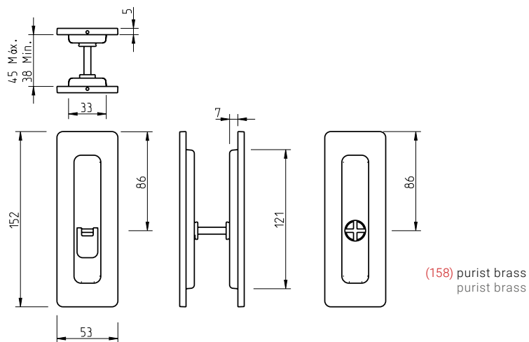
Asa de embutir - ENTRADA WC Flush handle - WC ENTRY
