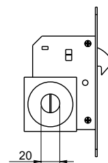
Fechadura para portas de correr Sliding doors locks
