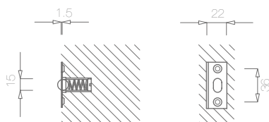
Fecho de esfera Recomendado para janelas de porta
