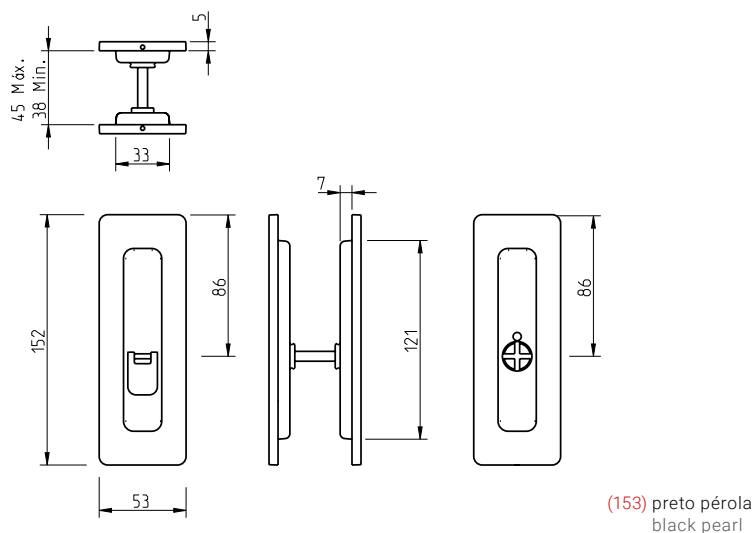
Asa de embutir - ENTRADA WC Livre/Ocupado Flush handle - Free/Occupied WC ENTRY
